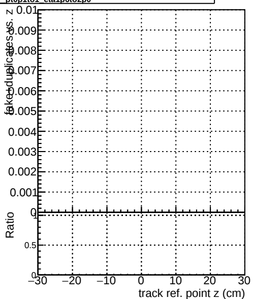
pt0p1to1-eta106to200 pt0p1to1-eta106to200 pt0p1to1-eta106to200
