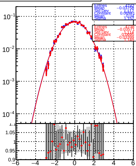
RecoPVAssoc2GenPVMatched_PulIZ
