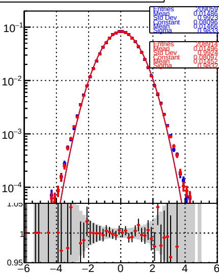
RecoAllAssoc2GenMatched_PulIX
