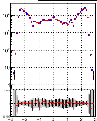
—●— DQM_TT_mkFit-DQM —●— DQM_TT_mkFitRETEST-DQM
