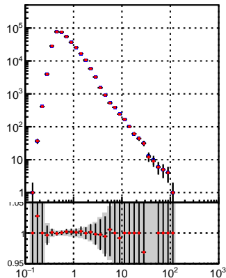
—●— DQM_TT_mkFit-DQM —●— DQM_TT_mkFitRETEST-DQM
