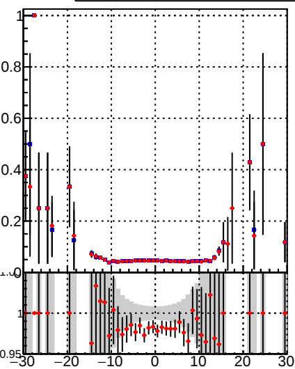
■ DQM_TT_mkFit-DQM_ ● DQM_TT_mkFitRETEST-DQM_
