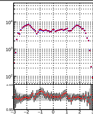
DQM_TT_mkFit-DQM DQM_TT_mkFitRETEST-DQM
