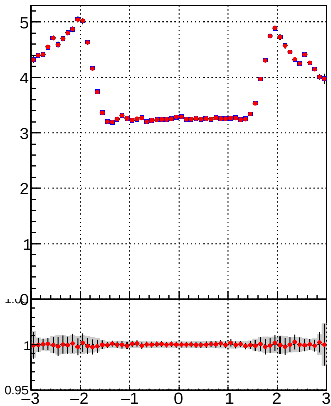
— DQM_TT_mkFit-DQM_ — DQM_TT_mkFitRETEST-DQM_
