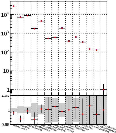
Number —●— DQM_TT_mkFitRETEST-DQM
