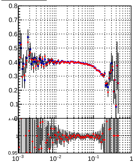
■ DQM_TT_mkFit-DQM_ ● DQM_TT_mkFitRETEST-DQM_
