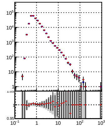
DQM_TT_mkFit-DQM DQM_TT_mkFitRETEST-DQM_
