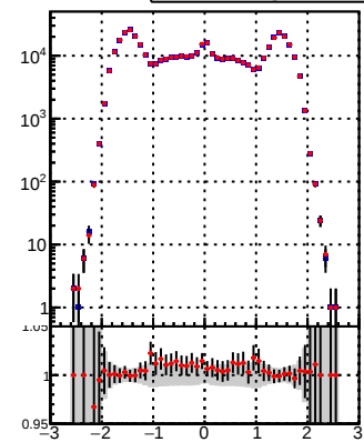
DQM_TT_mkFit-DQM DQM_TT_mkFitRETEST-DQM_
