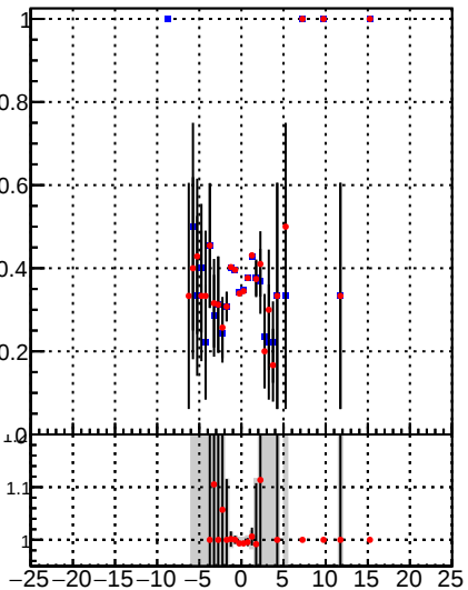
Fake rate vs d —●— DQM TT mkFit-DQM —●— DQM TT mkFitRETEST-DQM
