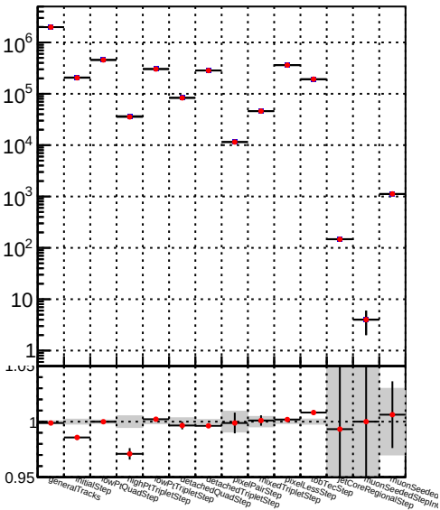
Number —●— DQM_TT_mkFitRETEST3
