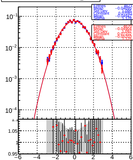
RecoPVAssoc2GenPVMatched_PulIZ
