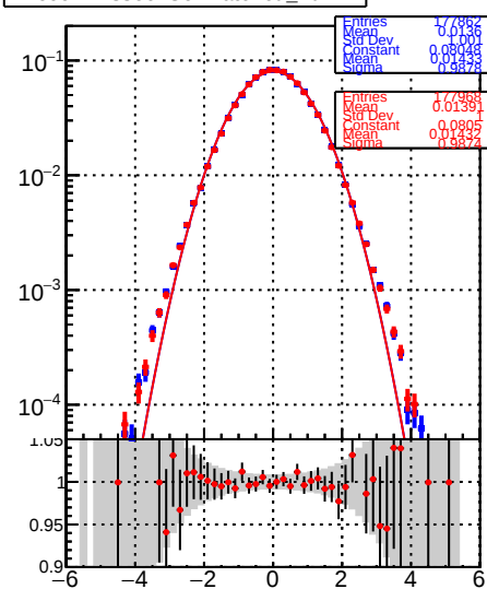
RecoAllAssoc2GenMatched_PulIX
