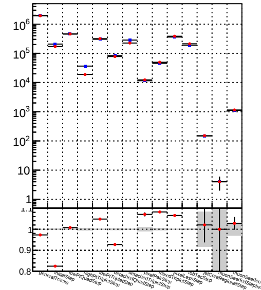
Number —●— DQM_TT__mkFitRETEST2_
