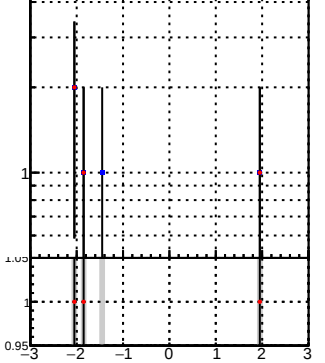
N of reco track vs eta
