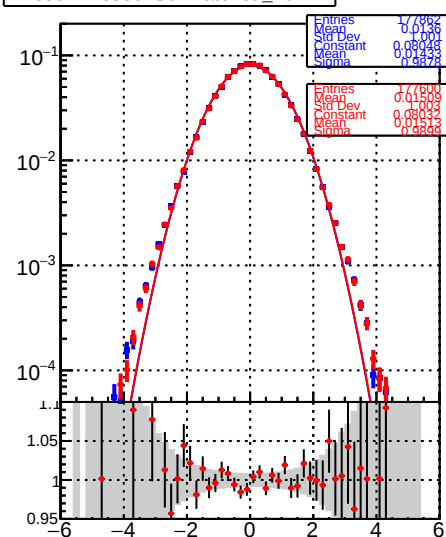
RecoAllAssoc2GenMatched_PulIX
