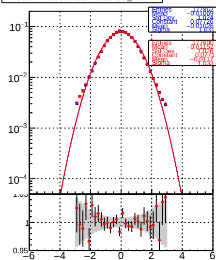
RecoAllAssoc2GenMatched_PulIZ
