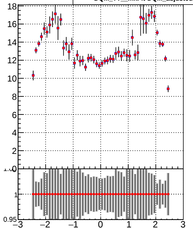
mean # STRIP hits vs eta
