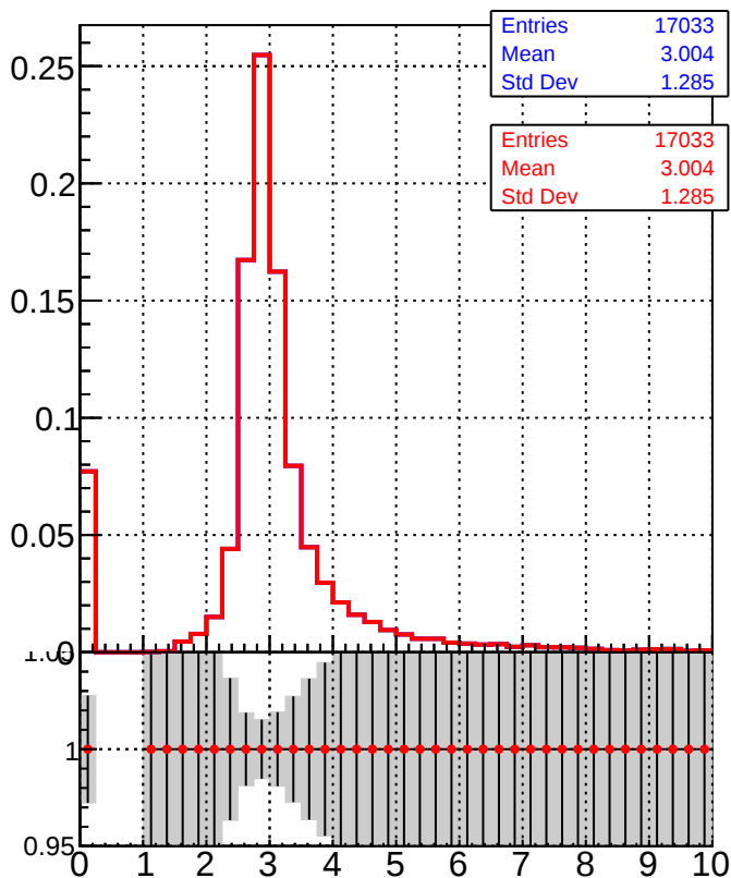
dE/dx estimator 2
