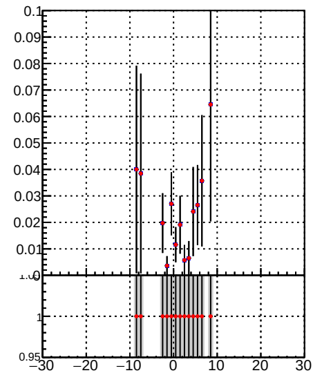
—•— DQM TT mkFit-DQM_i2 —•— DQM TT mkFit-DQM_adjustedi2
