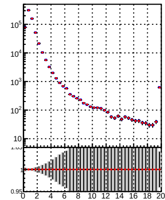
Legend: DQM TT mkFit-DQM i2 DQM TT mkFit-DQM adjustedi2 verSet
