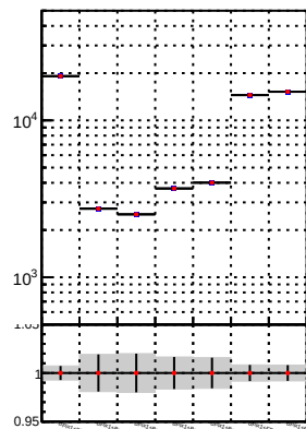
Legend: DQM TT mkFit-DQM i2 DQM TT mkFit-DQM adjustedi2 verSet
