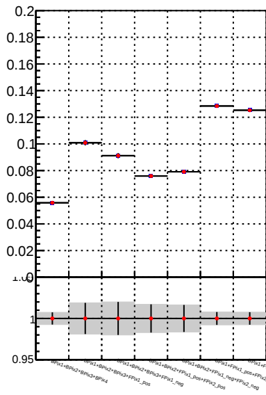
Fake rate vs. DQM TT mkFit-DQM i2 DQM TT mkFit-DQM adjustedi2
