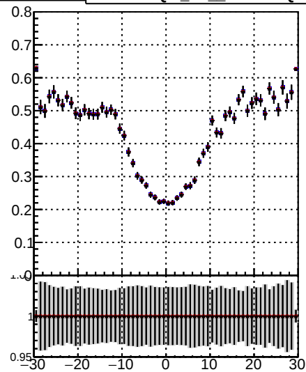
—•— DQM TT mkFit-DQM —•— DQM TT mkFit-DQM adjusted —•— DQM TT mkFit-DQM adjusted2
