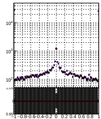
—•— DQM TT mkFit-DQM —•— DQM TT mkFit-DQM adjusted —•— DQM TT mkFit-DQM adjustedi2
