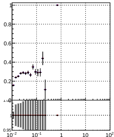
Fake rate vs vertpos Legend: DQM TT mkFit-DQM, DQM TT mkFit-DQM adjusted, DQM TT mkFit-DQM adjusted2
