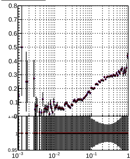
Fake rate vs \sqrt{s} DQM TT mkFit-DQM DQM TT mkFit-DQM adjusted DQM TT mkFit-DQM adjusted2
