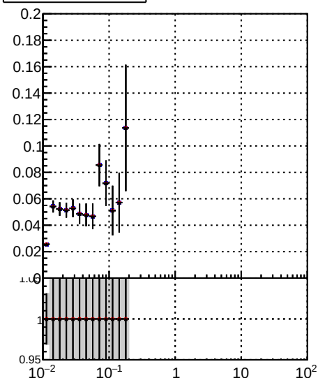
—●— DQM TT mkFit-DQM —●— DQM TT mkFit-DQM adjusted2 —●— DQM TT mkFit-DQM adjusted2
