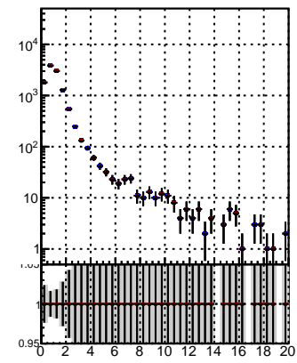
N of reco track vs. \chi^2 \chi^2 bin BQM TT mkFit-BQM adjusted 0-2 ~10^3 ~10^3 ~10^3 2-4 ~10^3 ~10^3 ~10^3 4-6 ~10^3 ~10^3 ~10^3 6-8 ~10^3 ~10^3 ~10^3 8-10 ~10^3 ~10^3 ~10^3 10-12 ~10^3 ~10^3 ~10^3 12-14 ~10^3 ~10^3 ~10^3 14-16 ~10^3 ~10^3 ~10^3 16-18 ~10^3 ~10^3 ~10^3 18-20 ~10^3 ~10^3 ~10^3
