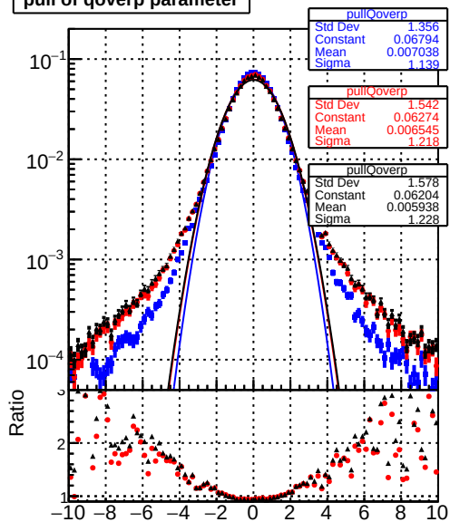
pull of qoverp parameter
