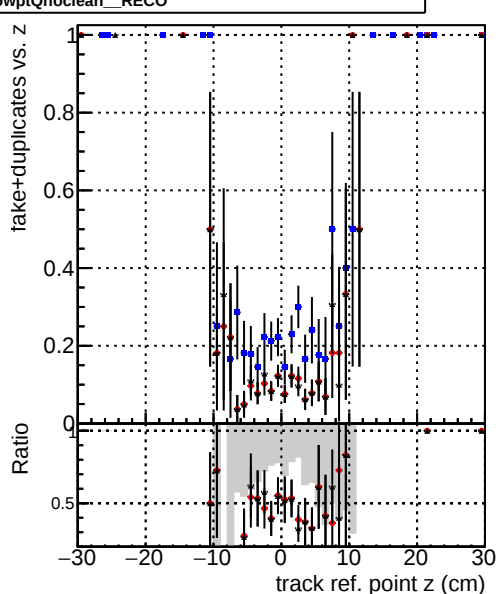
FitPU50LowPtQuad__RECO ptOnoclean__RECO
