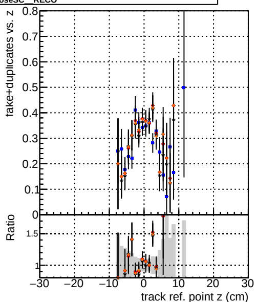
ptQnoclean__RECO eSC__RECO
