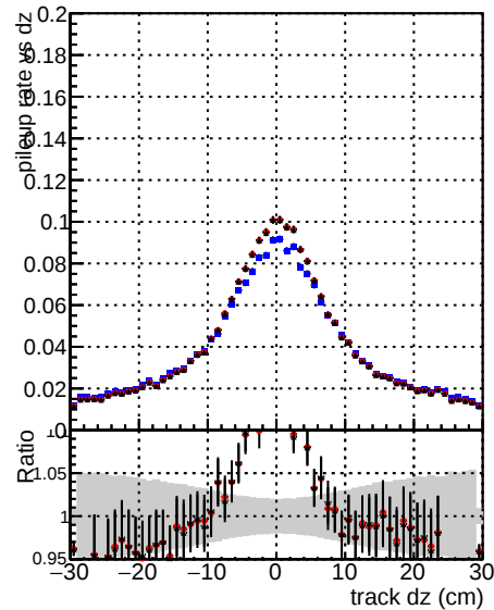
Global CMSSW ckfPU50 RECO Global CMSSW InFPU50LowPtQuad RECO Global CMSSW LowPtOnClean RECO
