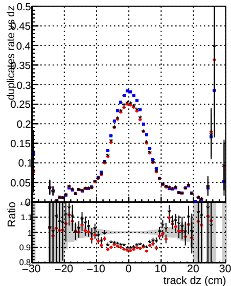
Global CMSSW ckfPU50 RECO Global CMSSW ckfPU50 LowPtQuad RECO
