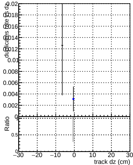
mkFitPU50LowptOnoc
