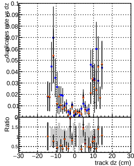
LowBtOnoSC-RECCO
