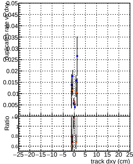
LowBtOnoSC-RECCO
