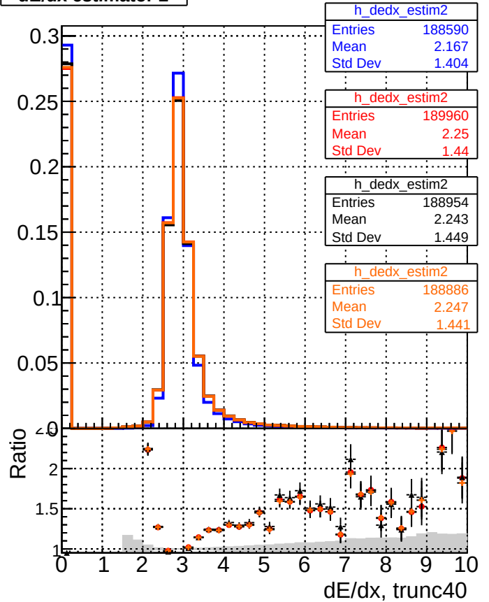
dE/dx estimator 2
