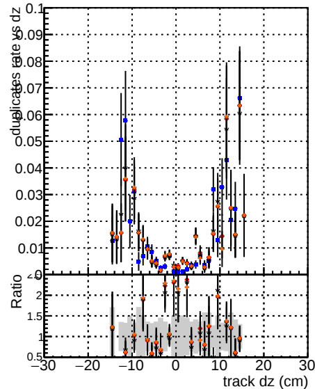
CMSSW LowptOnDC-RECO
