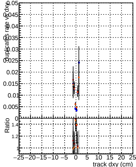
CMSSW LowptOnDC-RECO
