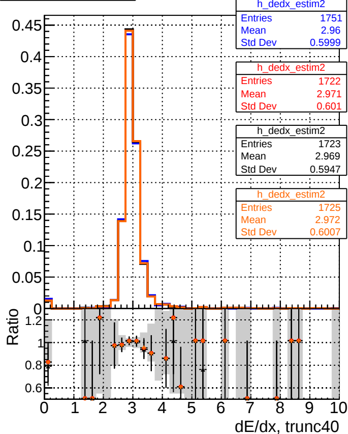
dE/dx estimator 2
