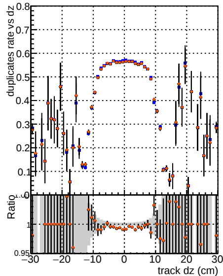
CMSSW-HKFiTPU50E8
