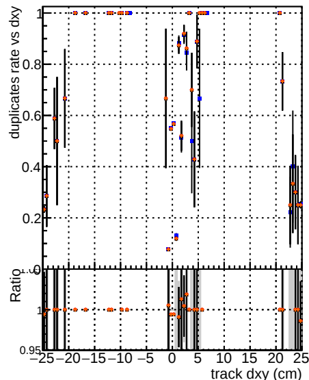
CMSSW-HKFiTPU50E8
