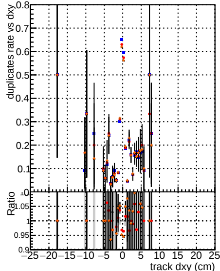
CMSSW-MkFitPU50E8
