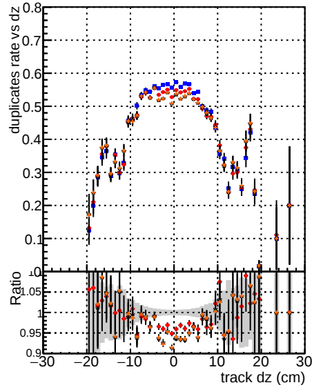
CMSSW-MkFitPU50E8
