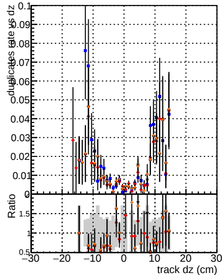
CMMSWWHKKTTTTpU50LowPtoQuad RECO CMMSWWHKKTTTTpU50LowPtoQuad-noBkwd RECO
