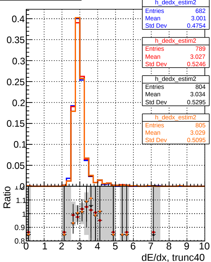
dE/dx estimator 2
