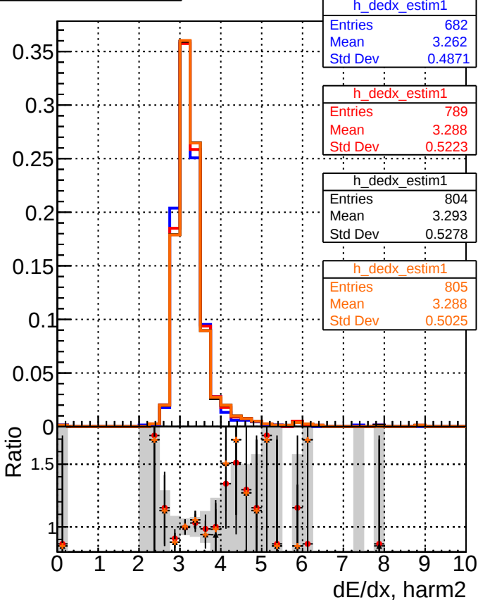
dE/dx estimator 1
