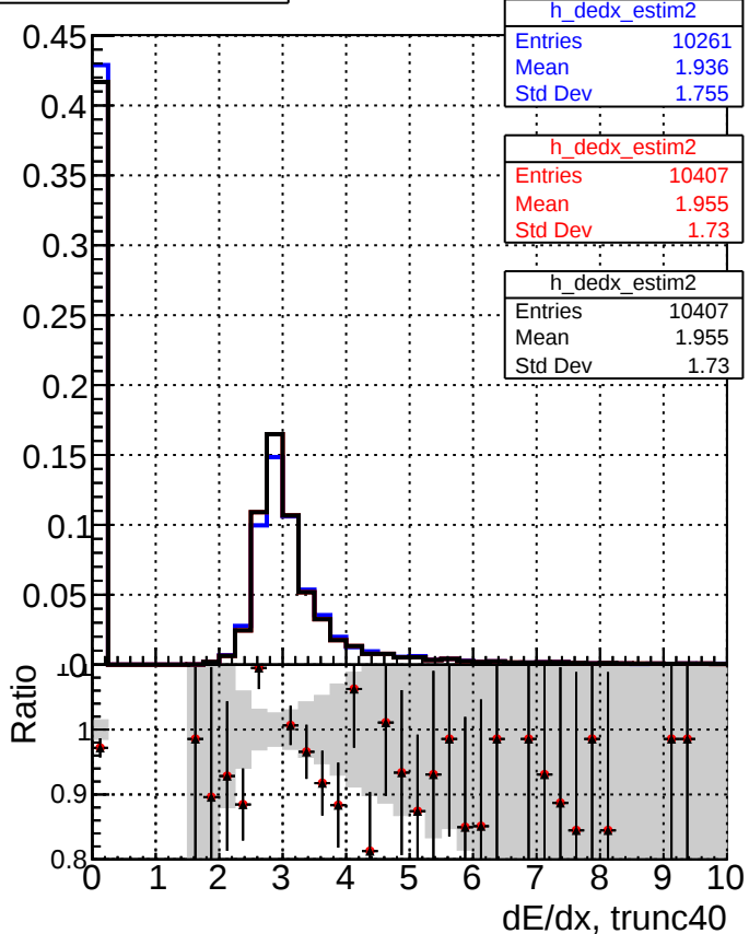
dE/dx estimator 2
