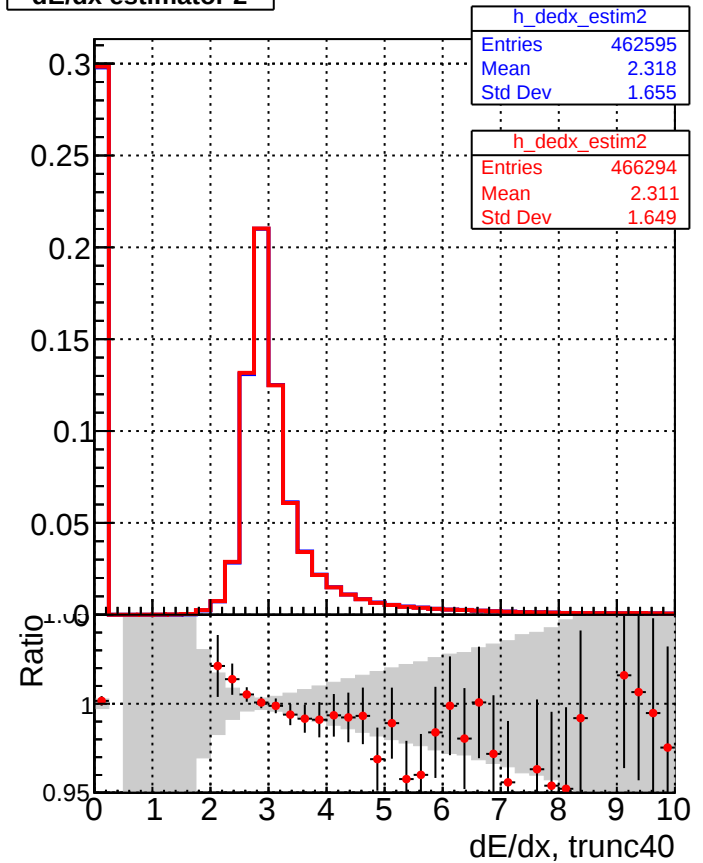
dE/dx estimator 2
