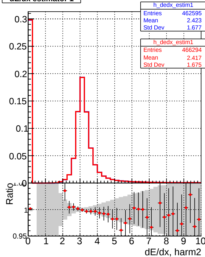
dE/dx estimator 1
