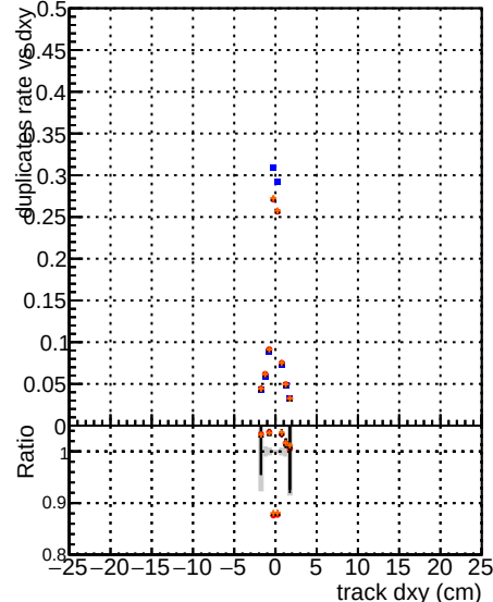
05+dup RECO
