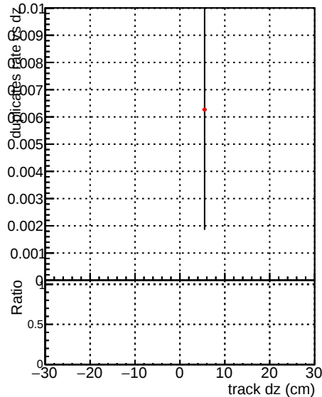
CMSSW-HKFitPU50LowPtQuad RECO CMSSW-HKFitPU50LowPtTriplet RECO
