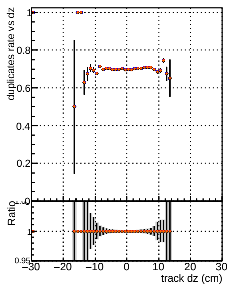
al=CMSSW-MkfitLowPtQuad-RECO al=CMSSW-MkfitLowPtTriplet-RECO
