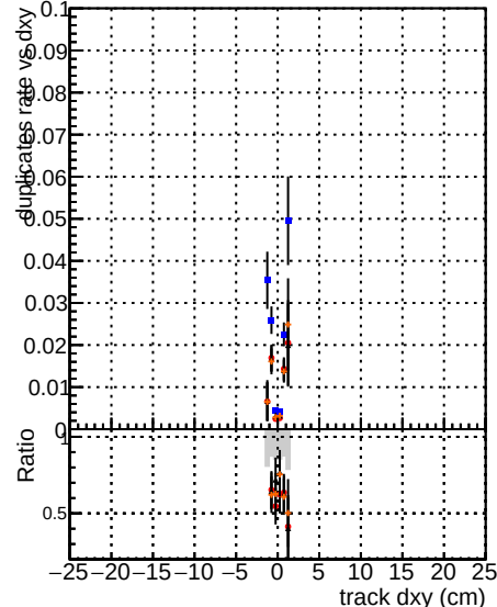
CMSSW HkfltLowPtQuad RECO CMSSW HkfltLowPtTriplet RECO
