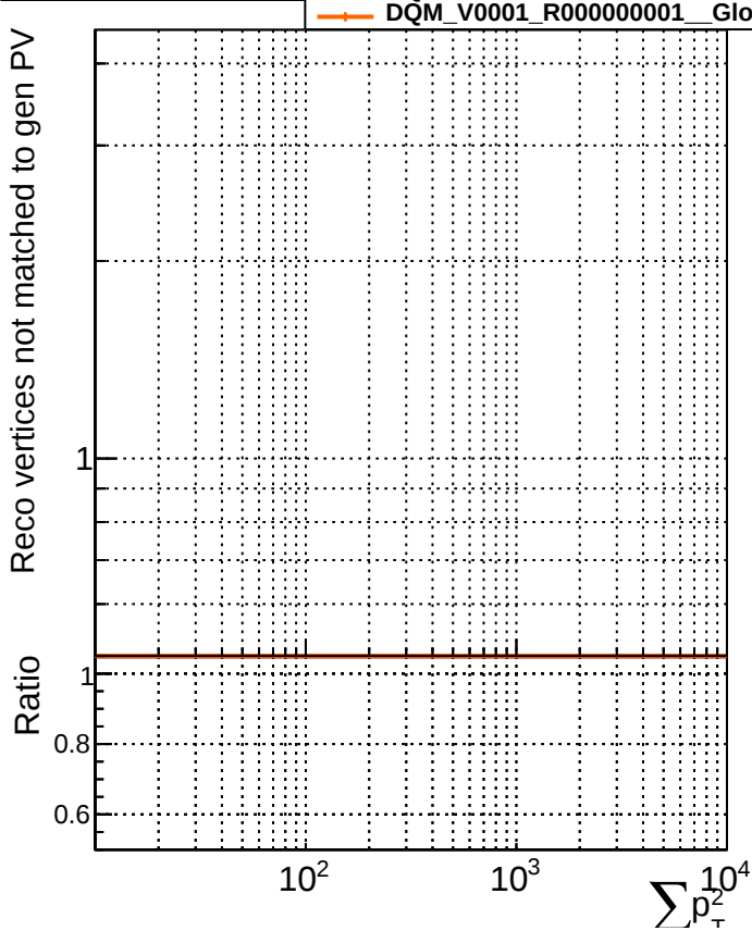
RecoAssoc2GenPV
