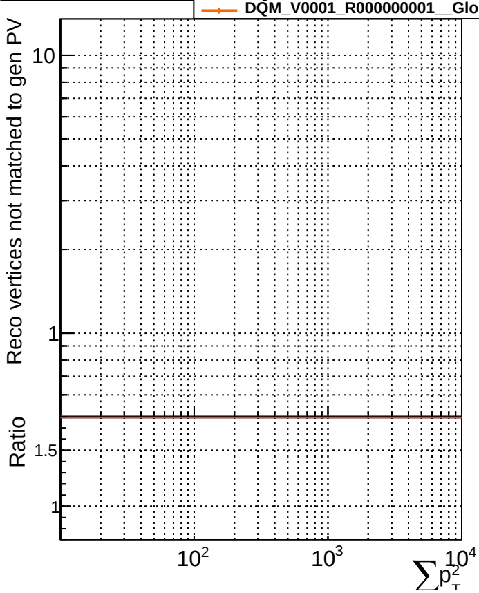
RecoAssoc2GenPV
