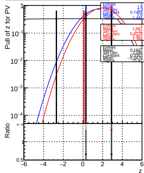
RecoPVAssoc2GenPVMatched_PullZ
