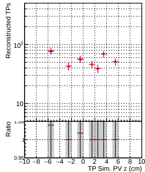
N of associated tracks (simToReco) vs. sim PV z 0 1 2 3 4 5 6 7 8 9 10 11 12 13 14 15 16 17 18 19 20 21 22 23 24 25 26 27 28 29 30 31 32 33 34 35 36 37 38 39 40 41 42 43 44 45 46 47 48 49 50 51 52 53 54 55 56 57 58 59 60 61 62 63 64 65 66 67 68 69 70 71 72 73 74 75 76 77 78 79 80 81 82 83 84 85 86 87 88 89 90 91 92 93 94 95 96 97 98 99 100 101 102 103 104 105 106 107 108 109 110 111 112 113 114 115 116 117 118 119 120 121 122 123 124 125 126 127 128 129 130 131 132 133 134 135 136 137 138 139 140 141 142 143 144 145 146 147 148 149 150 151 152 153 154 155 156 157 158 159 160 161 162 163 164 165 166 167 168 169 170 171 172 173 174 175 176 177 178 179 180 181 182 183 184 185 186 187 188 189 190 191 192 193 194 195 196 197 198 199 200 201 202 203 204 205 206 207 208 209 210 211 212 213 214 215 216 217 218 219 220 221 222 223 224 225 226 227 228 229 230 231 232 233 234 235 236 237 238 239 240 241 242 243 244 245 246 247 248 249 250 251 252 253 254 255 256 257 258 259 260 261 262 263 264 265 266 267 268 269 270 271 272 273 274 275 276 277 278 279 280 281 282 283 284 285 286 287 288 289 290 291 292 293 294 295 296 297 298 299 300 301 302 303 304 305 306 307 308 309 310 311 312 313 314 315 316 317 318 319 320 321 322 323 324 325 326 327 328 329 330 331 332</
